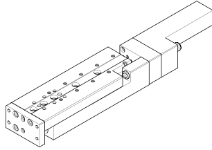
Mini slide EGSC-BS-KF-...
