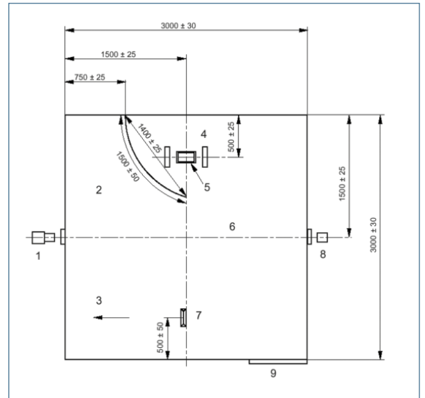
Duman yoğunluğu test kabini, yerleşim planı.
