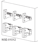
Düsey Bara Bağlantı Parçaları
